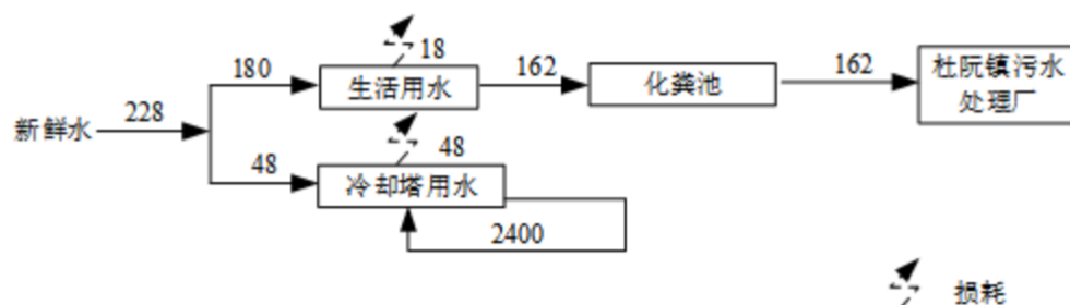
图 1. 迁扩建后全厂水平衡图 (t/a)
