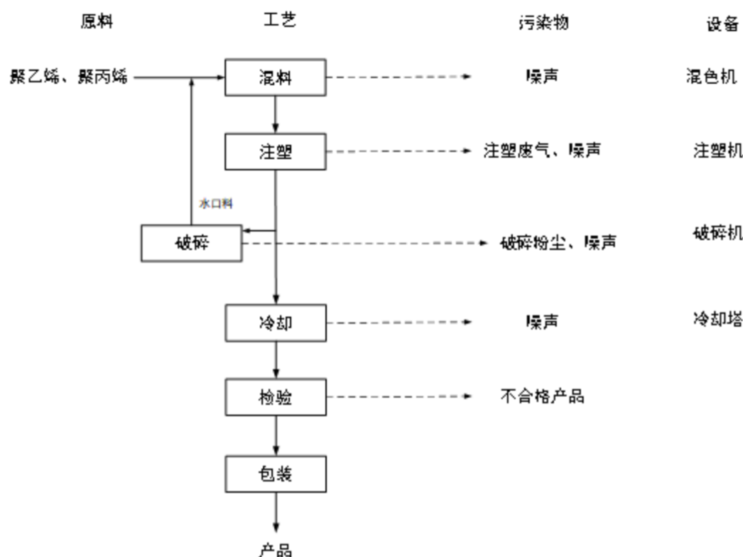
图3. 生产工艺流程图
