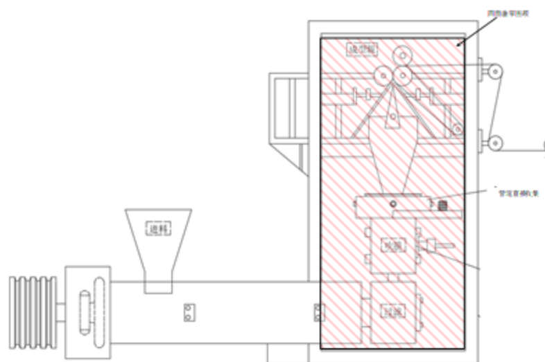
图 4-2 吹膜装置收集示意图
