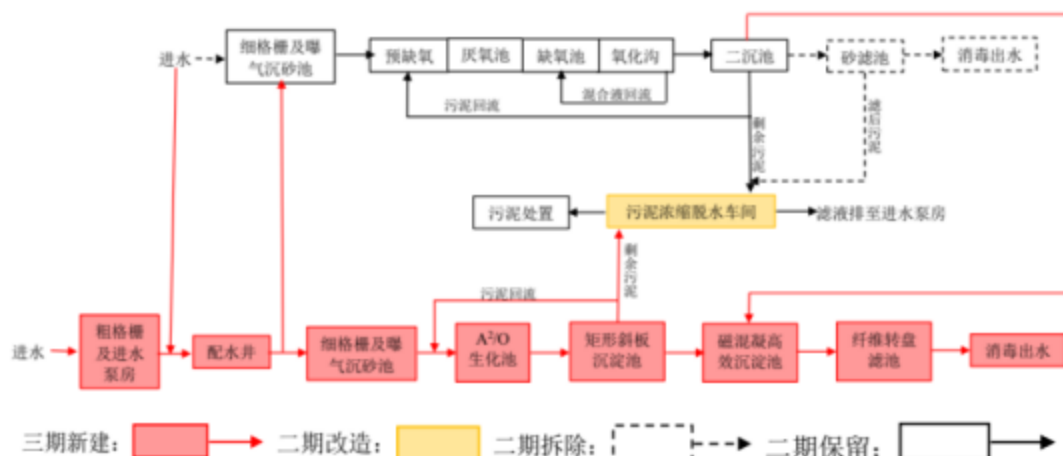
图 4-4 荷塘镇生活污水处理厂工艺流程图
