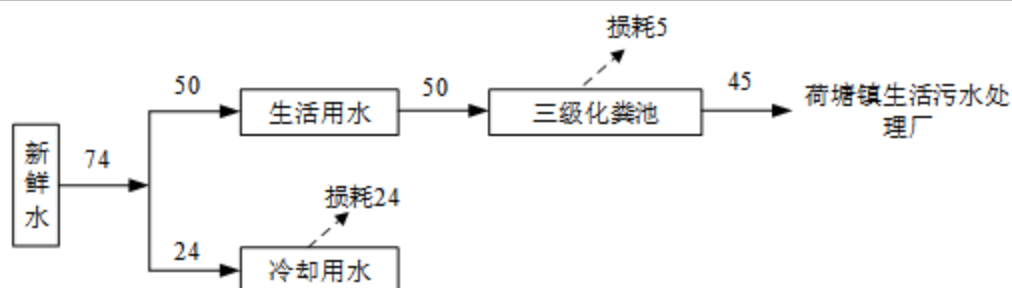
图 2-1 项目水平衡图 (t/a)
