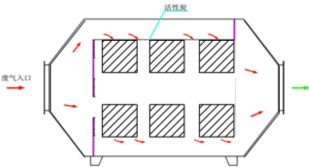
图 4.3 活性炭装置结构示意图
